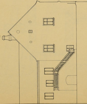
PÉCS Kardoss Kálmán u. B sz. 2866-97 ház.
